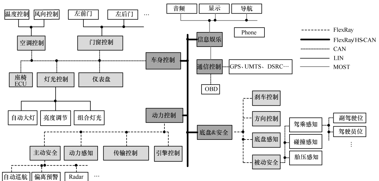
图2 一种典型的车载网络结构
